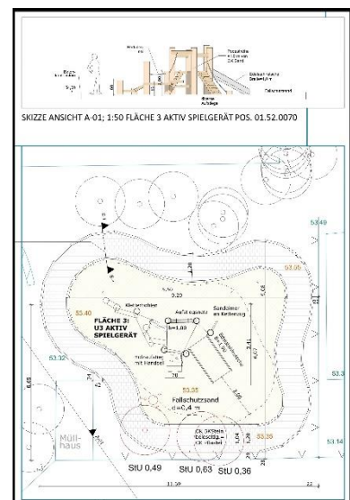
Ausschnitt aus der Ausführungsplanung (Grafik: bwgt e.V.)
